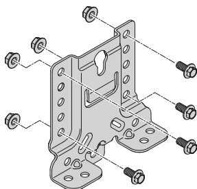
Крепление 4 винтами
