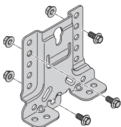
Крепление 3 винтами
